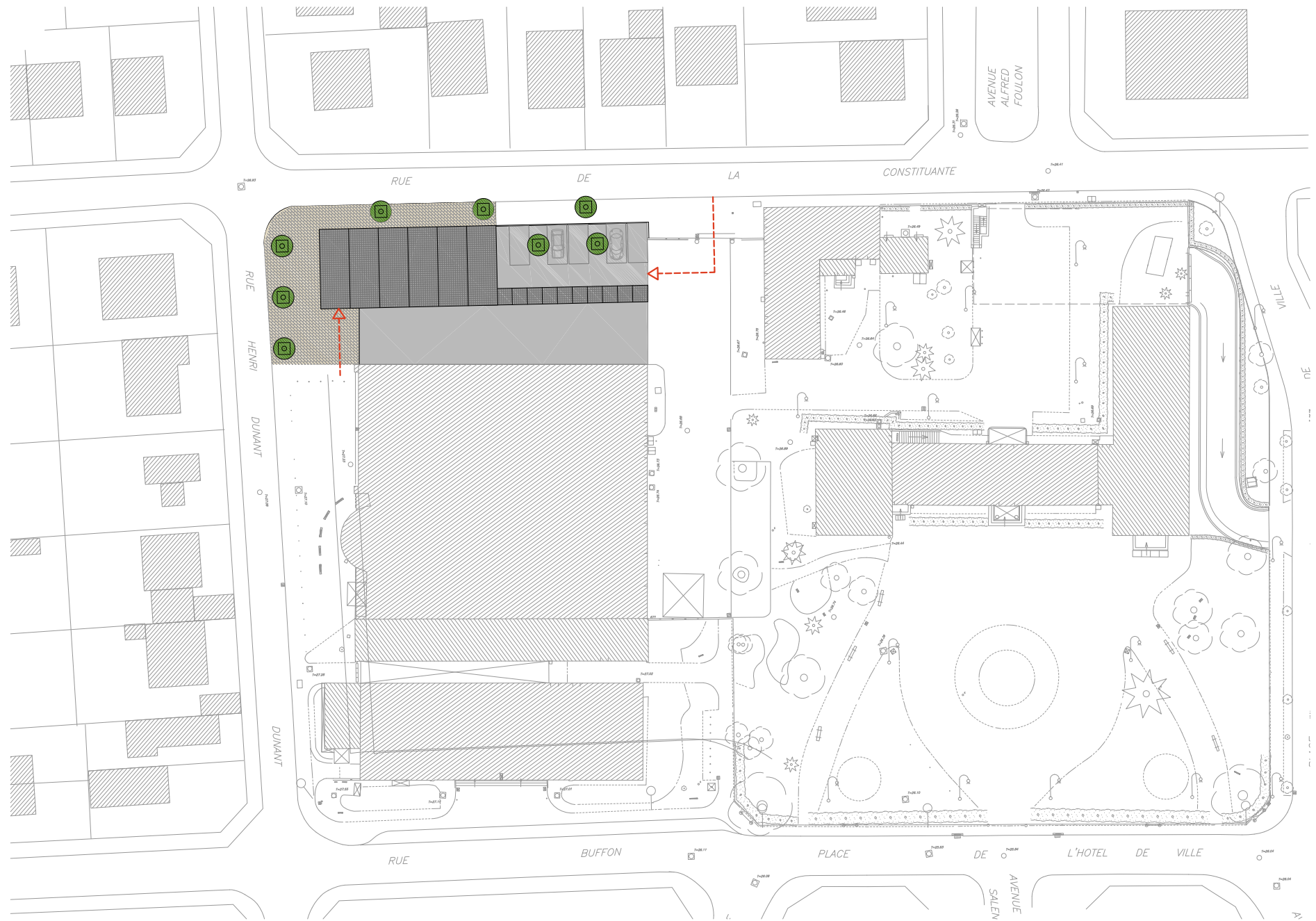
PLAN MASSE - échelle : 1/1000°
